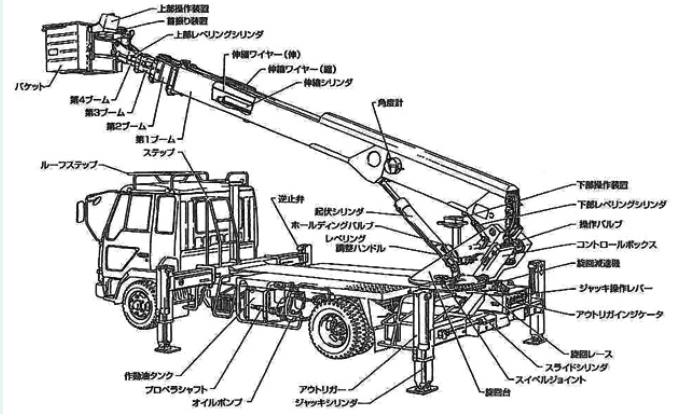
伸縮ブーム型高所作業車
